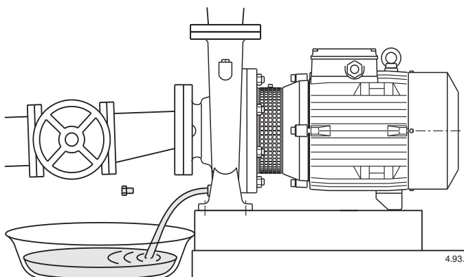
Рис. 4 Слив воды
